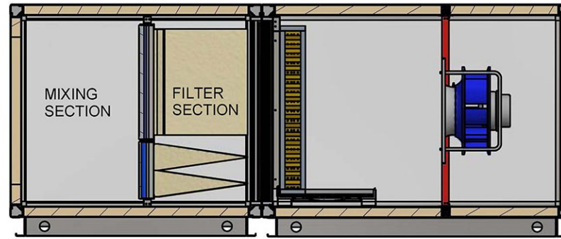
A-A (1 : 28)
